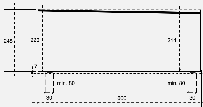
PRZEKRÓJ PODŁUŻNY
